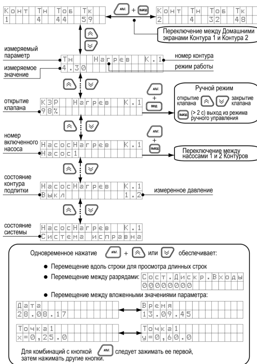
Рисунок 7.2 – Рабочие экраны 1
